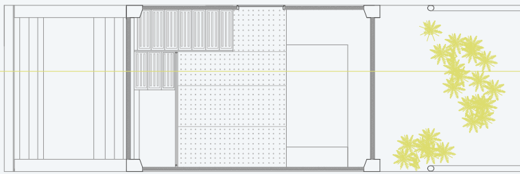
PLANTA SUPERIOR
